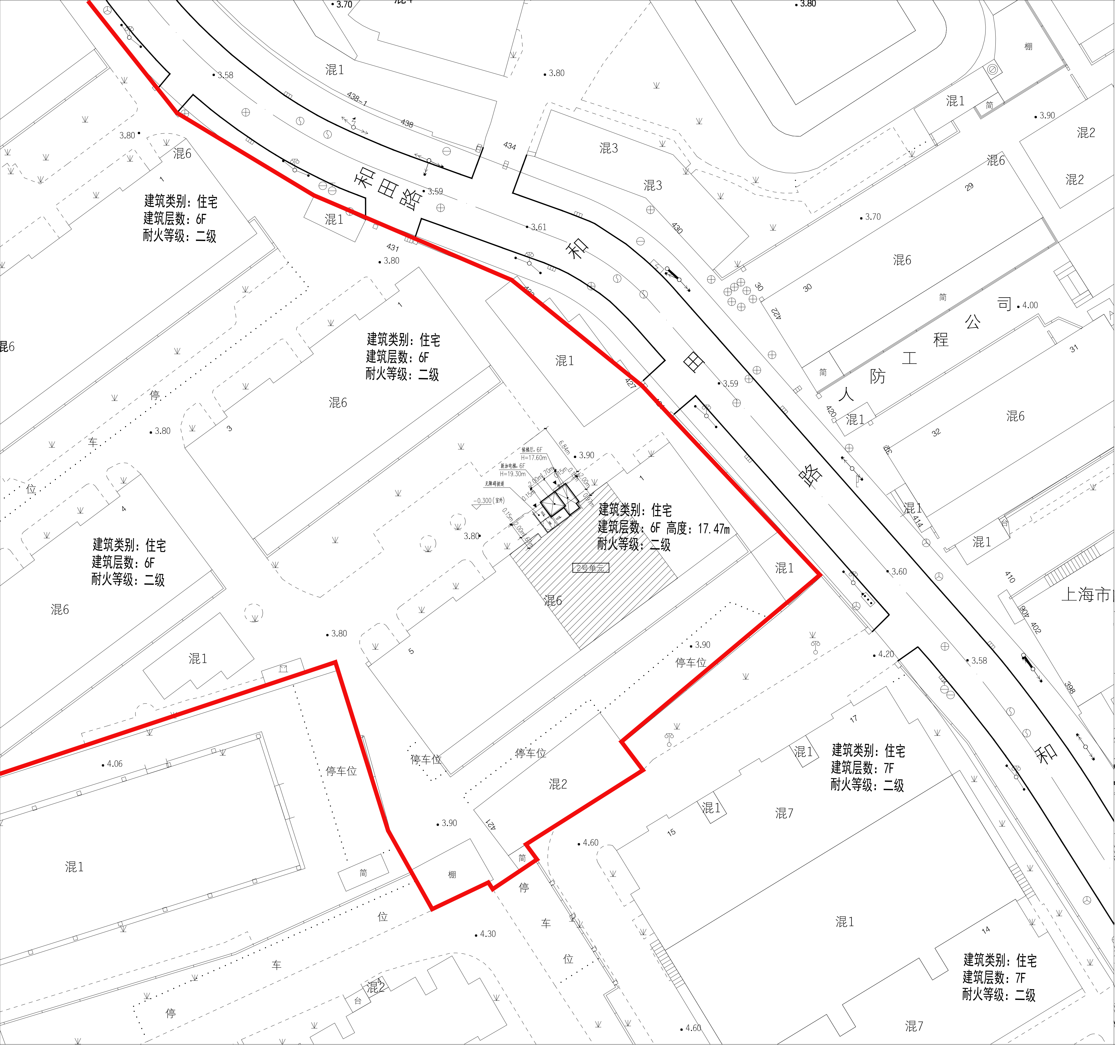
总平面图
