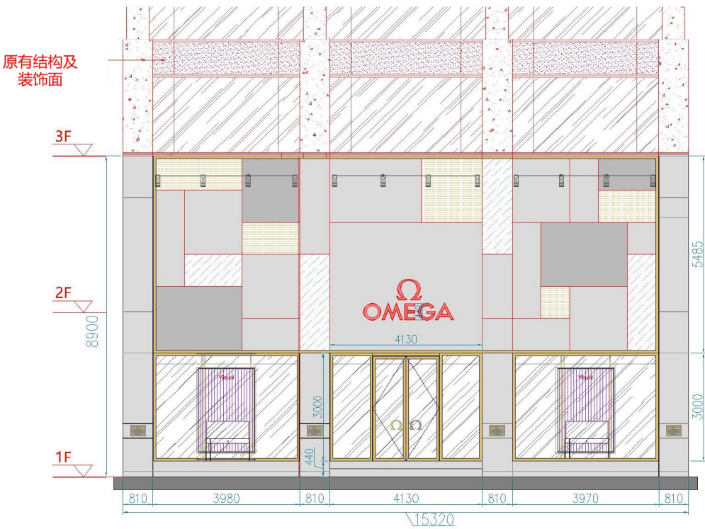
南京西路立面图
